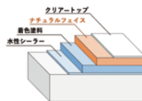
施工断面
