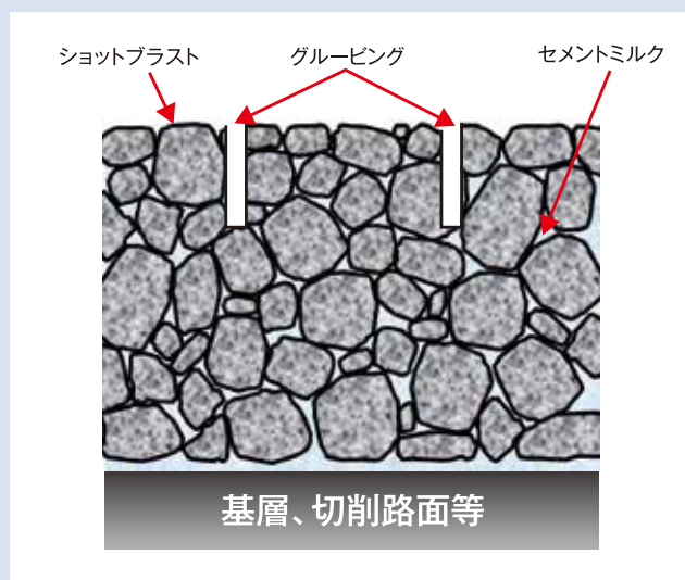
グルーブラストの構造イメージ
